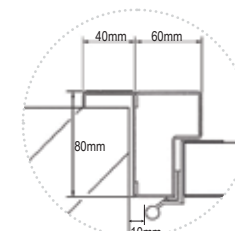
Dimensioni del telaio
